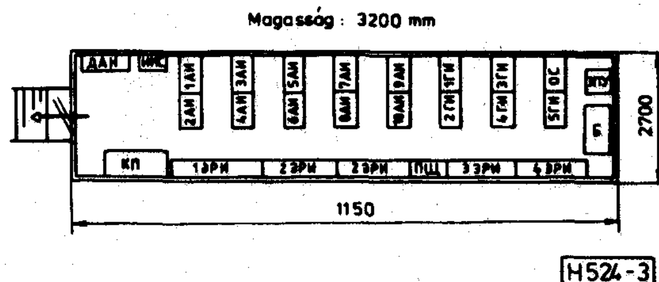
3. ábra. Konténeres ATSzK 100/2000 ER központ alaprajza
