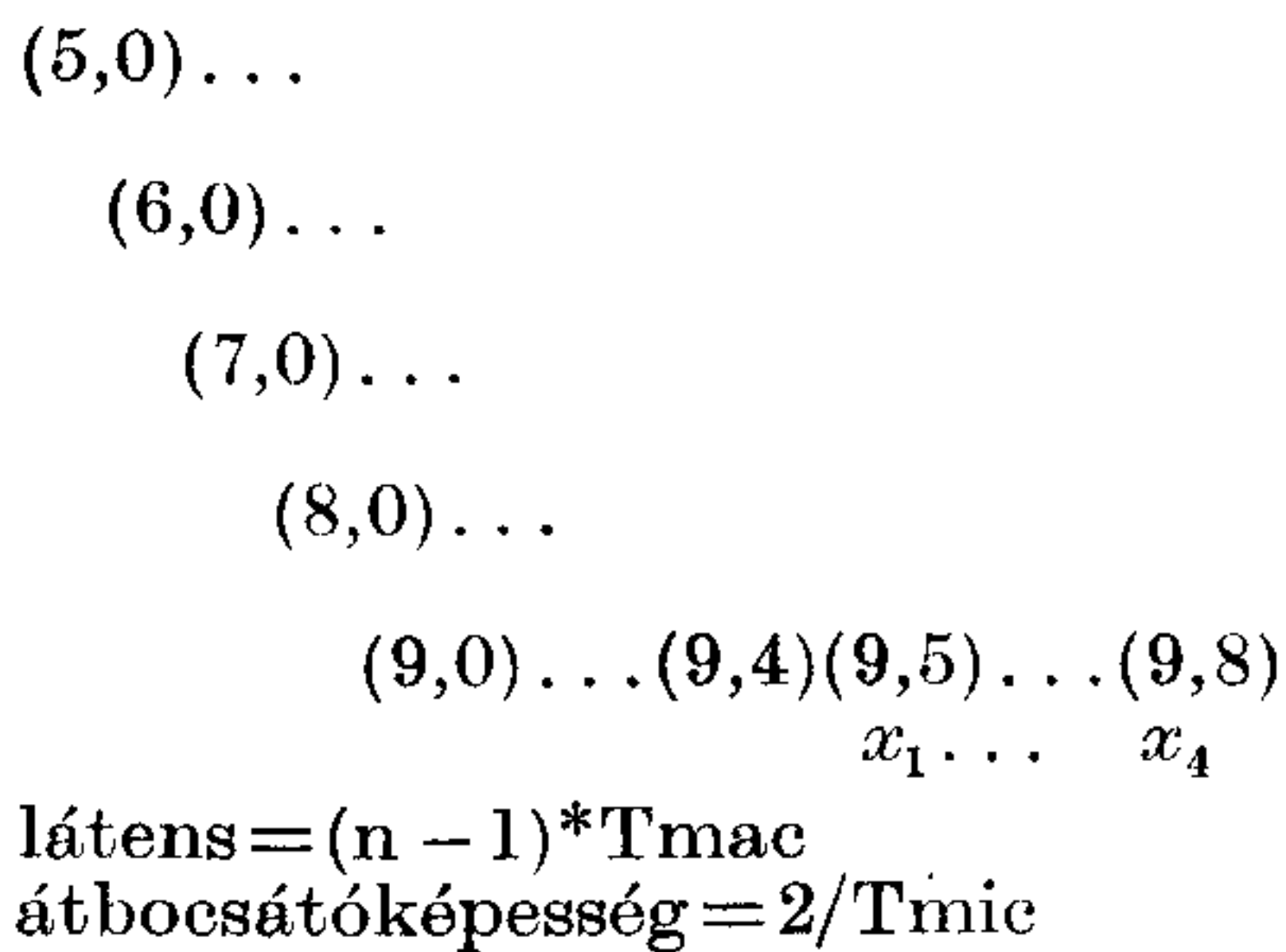
4. ábra. Lineáris egyenletrendszer CORDIC-proceszorok szisztolés tömbbel való megoldása
