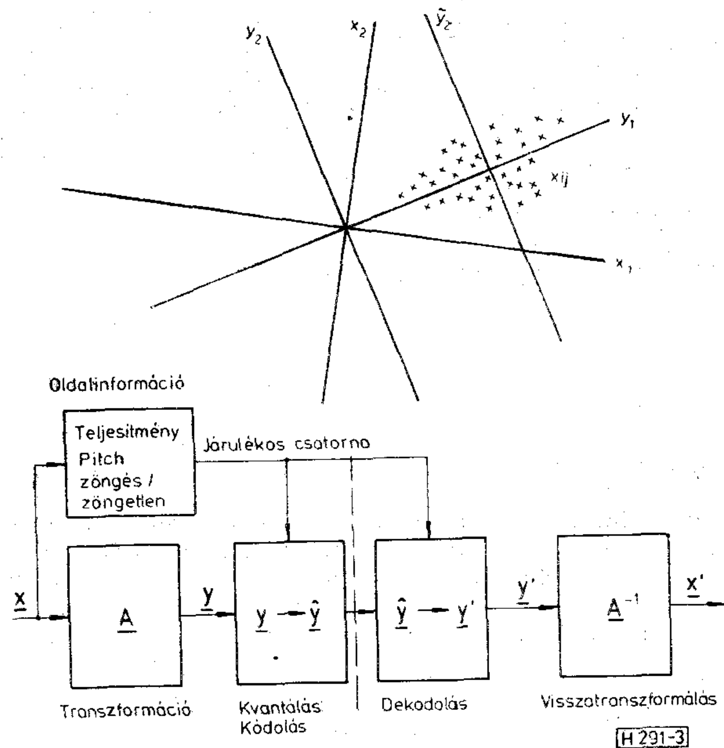
3. ábra. Transzformáció-kódoló; fent: koordinátatranszformáció; lent: elvi megvalósítás
