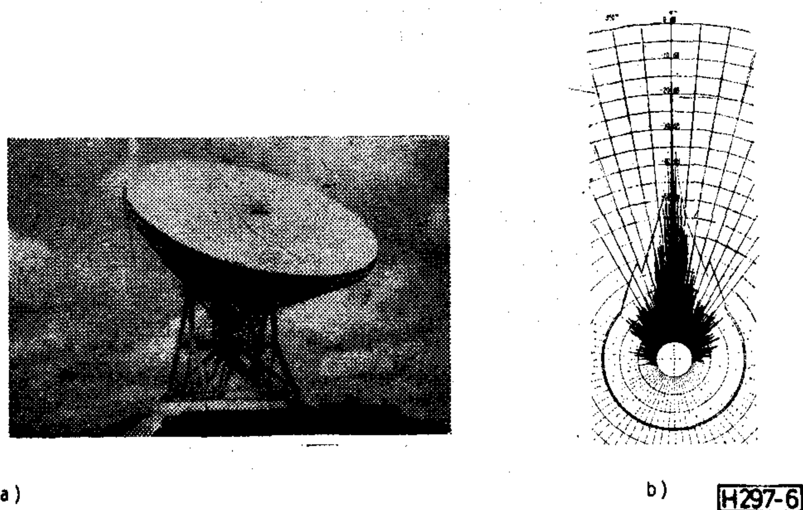
6. ábra. Burum 3 földi állomás (Hollandia. Foto: Siemens) a., Felépítése b., Iránykarakterisztika
