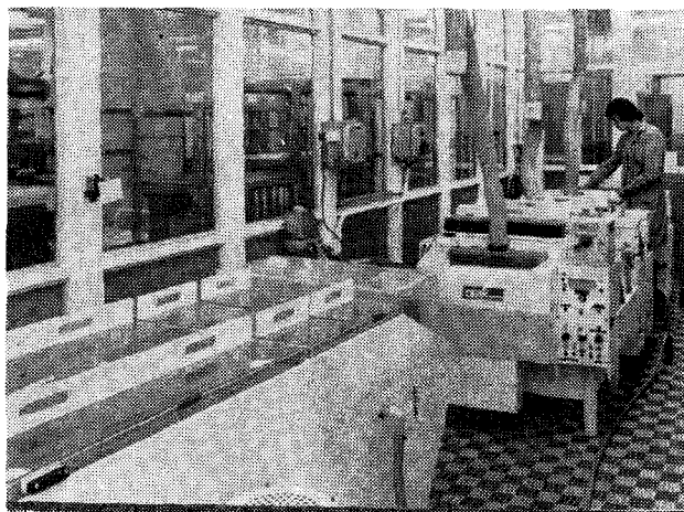
Előtérben a sztrippelőgép, mögötte a marató
