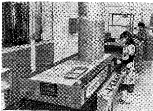
A nyáklap-gyártó üzem maratógépe
